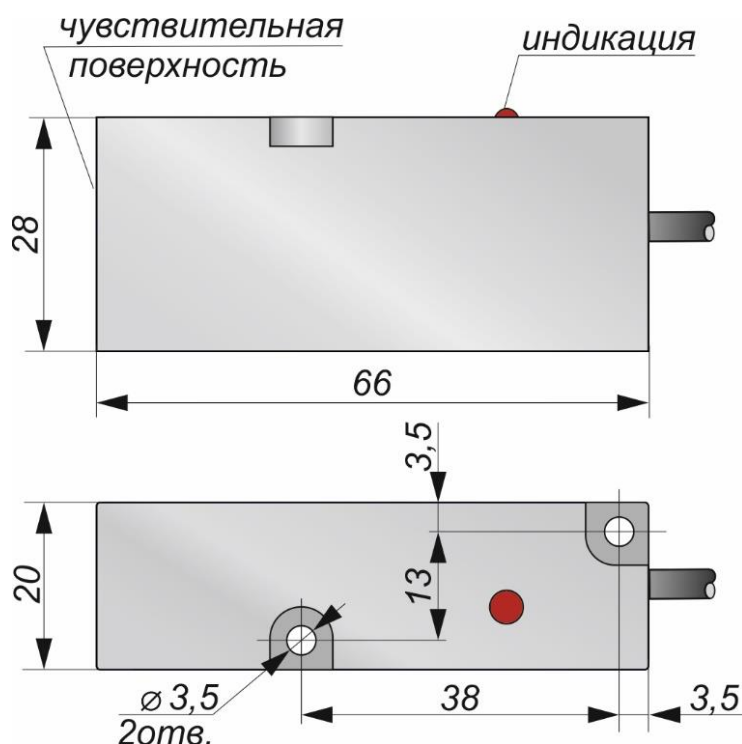
Габаритный чертеж
